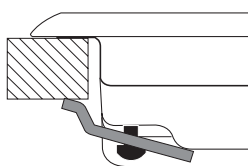
Poloha zaháknutia pre dosku H = 20 mm
