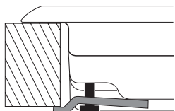
Poloha zaháknutia pre pracovnú dosku H = 40 mm
