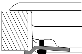
Posizione gancio per top H=40mm
