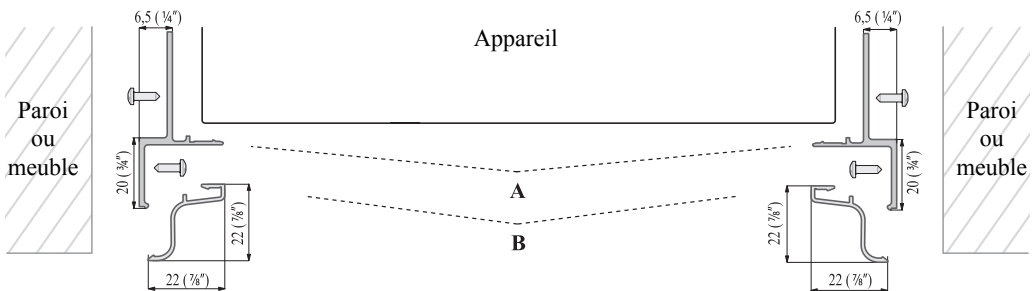
A Profil de raccordement
