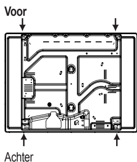
Stand haak voor keukenblad H=40mm
