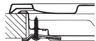
Posizione gancio per top H=30mm
