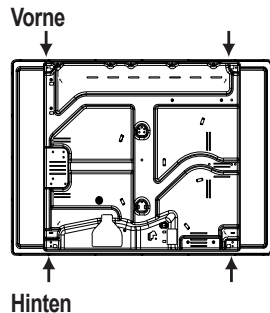
Position der Haken für Arbeitsplatten H=30mm
