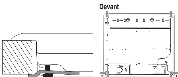
Position du crochet pour top H=40mm
