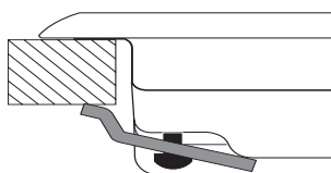
Розташування кріплення до стільниці Н=20mm
