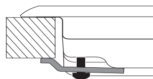
Stand haak voor keukenblad H=30mm
