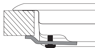
Розташування кріплення до стільниці Н=30mm
