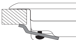
Position du crochet pour top H=20mm
