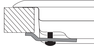
Posizione gancio per top H=30mm
