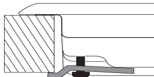
Posizione gancio per top H=40mm
