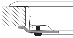
Position der Haken für Arbeitsplatten H=30mm
