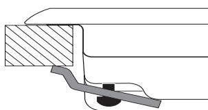
Stand haak voor keukenblad H=20mm
