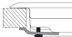
Position du crochet pour top H=30mm
