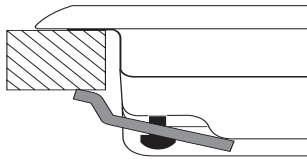
Position der Haken für Arbeitsplatten H=20mm
