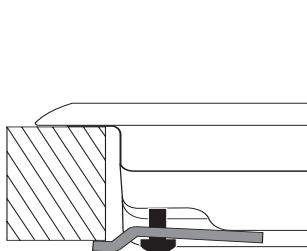
Position der Haken für Arbeitsplatten H=40mm
