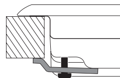
Posizione gancio per top H=30mm
