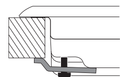
Position du crochet pour top H=30mm
