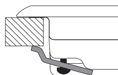
Position du crochet pour top H=20mm
