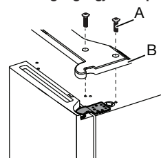
A. Skruvar övre gångjärnskåpa B. Övre gångjärnskåpa
