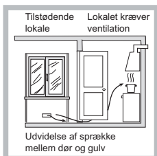
Eksempel på ventilationsåbninger til forbrændingsluft
