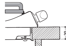
Placering af krog ved topstykke H=30mm
