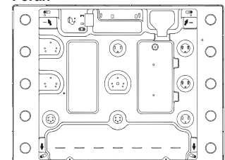
Placering af krog ved topstykke H=30mm
