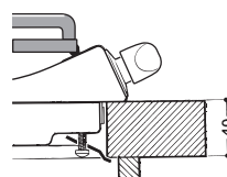
Placering af krog ved topstykke H=40mm
