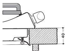
Position du crochet pour top H=40mm
