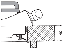
Position der Haken für Arbeitsplatten H=40mm
