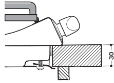
Position der Haken für Arbeitsplatten H=30mm
