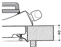
Stand haak voor keukenblad H=40mm
