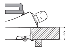
Stand haak voor keukenblad H=30\text{mm}
