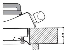
Posição do gancho para H=40mm
