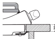
Position du crochet pour top H=20mm
