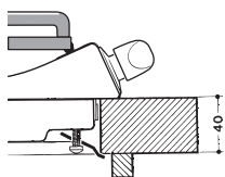
Posición del gancho para superficies H=40mm
