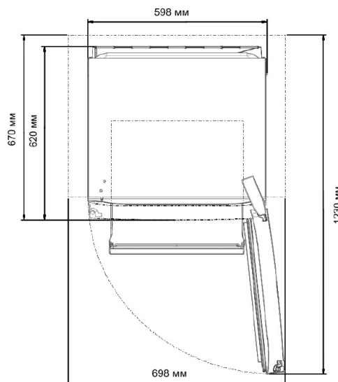
Робочі габарити холодильного приладу
